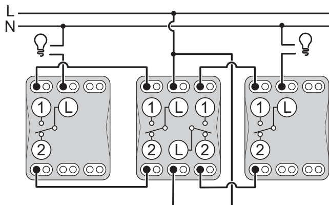
Kombinácia striedavých prepínačov s dvojítm striedavým prepínačom
