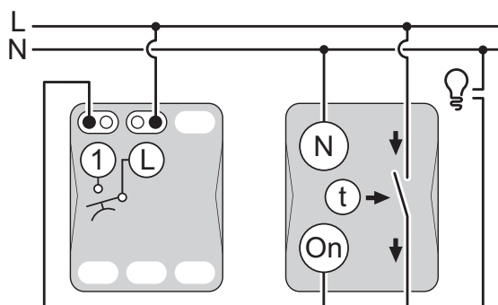
Ovládanie schodiskového svetla pomocou schodiskového časového spínača
