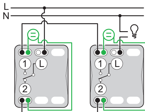
Dva striedavé prepínače (schodisková kombinácia) s orientačnou kontrolkou
