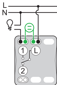
Jednopolové ovládanie zap/vyp s orientačnou kontrolkou
