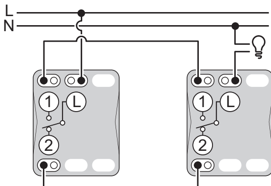
Dva striedavé prepínače (schodisková kombinácia)
