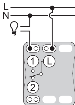
Jednopolové ovládanie zap/vyp
