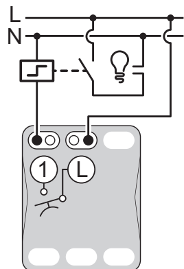
Ovládanie osvetlenia cez impulzné relé
