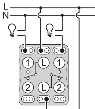
Dve jednopolové zap/vyp spínania
