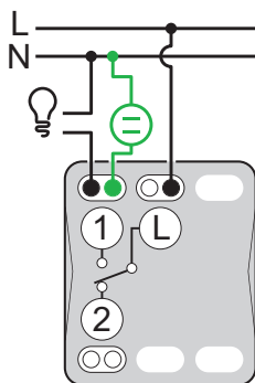
Jednopolové ovládanie zap/vyp so signalizačnou kontrolkou
