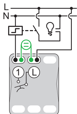
Ovládanie osvetlenia cez impulzné relé - orientačná kontrolka
