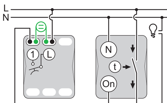
Ovládanie schodiskového svetla pomocou schodiskového časového spínača - orientačná kontrolka
